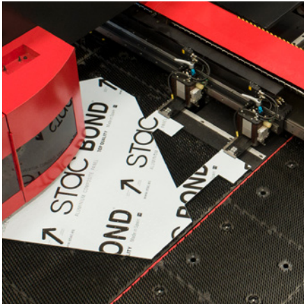
4 CNC pantographs 4 pantógrafos CNC 4 tables d'usinage CNC
